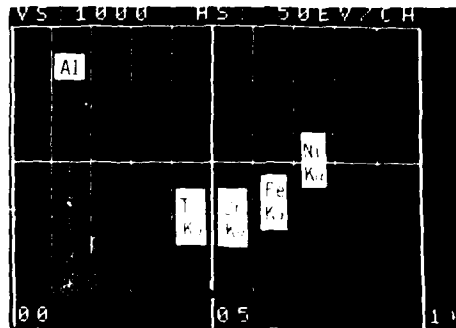
(d) Energy dispersive X-ray analysis of (c).
