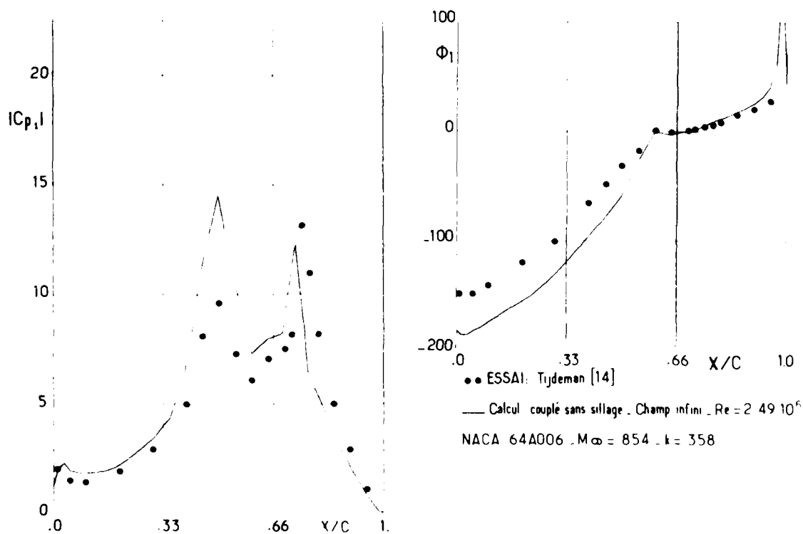
Fig. 10 : Champs des pressions instationnaires normalisées. Oscillation de gouverne 1°
