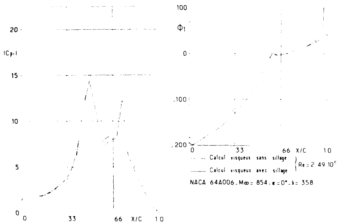
Fig. 12 : Champs des pressions instantanées, visualisés avec et sans prise en compte du sillage visqueux.
