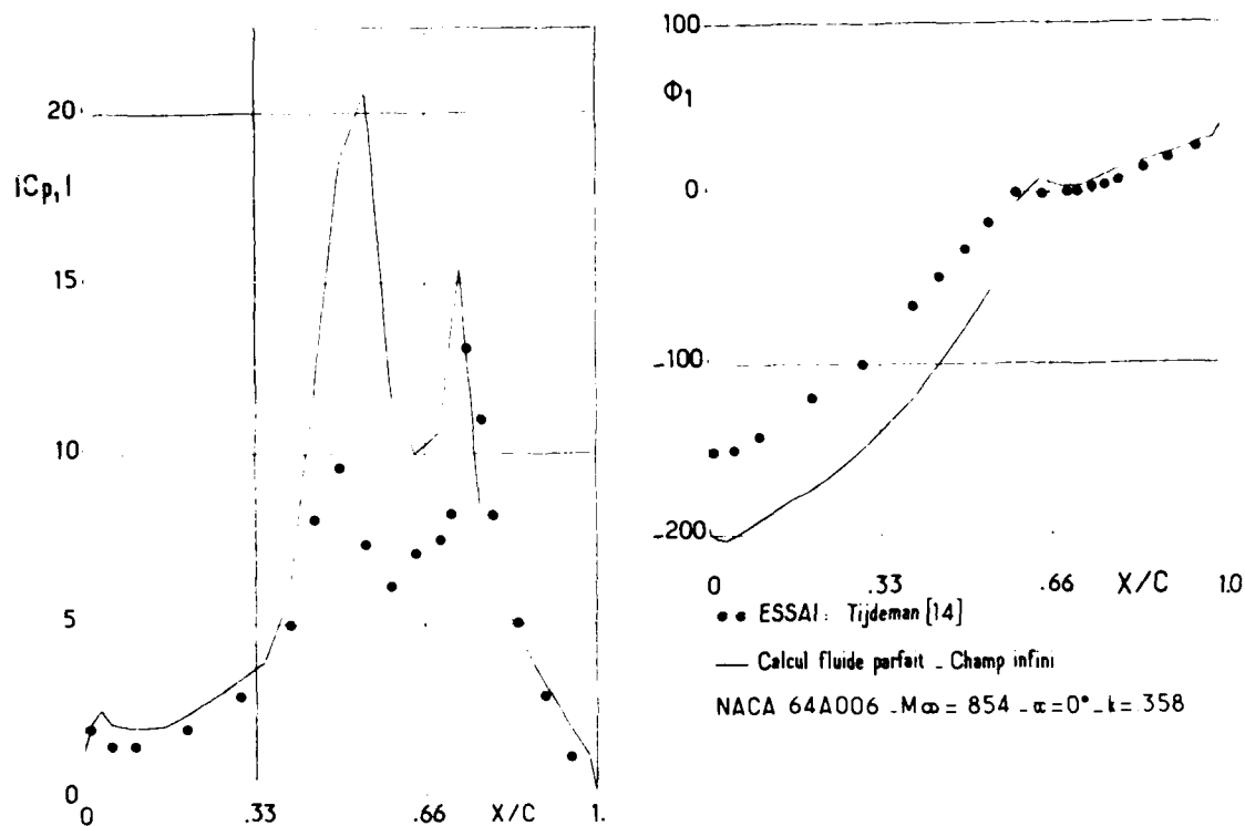
Fig. 9 : Champs des pressions instationnaires normalisées. Oscillation de gouverne 1°.
