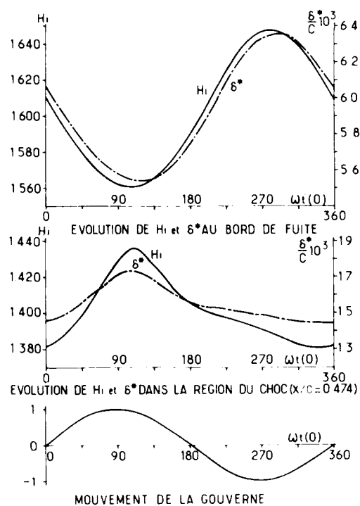
Fig. 13 : NACA 64 A 006 avec gouverne oscillante \alpha = 0,854 ; K = 0,358 ; \alpha = 0^\circ ; J_1 = 1^\circ ; Re = 2.49.10^6 .
