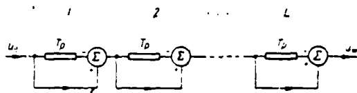
Fig. 8.1.6. L-fold subtraction system.
