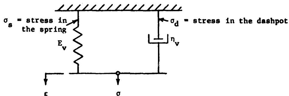
Figure 4. Voigt Model
