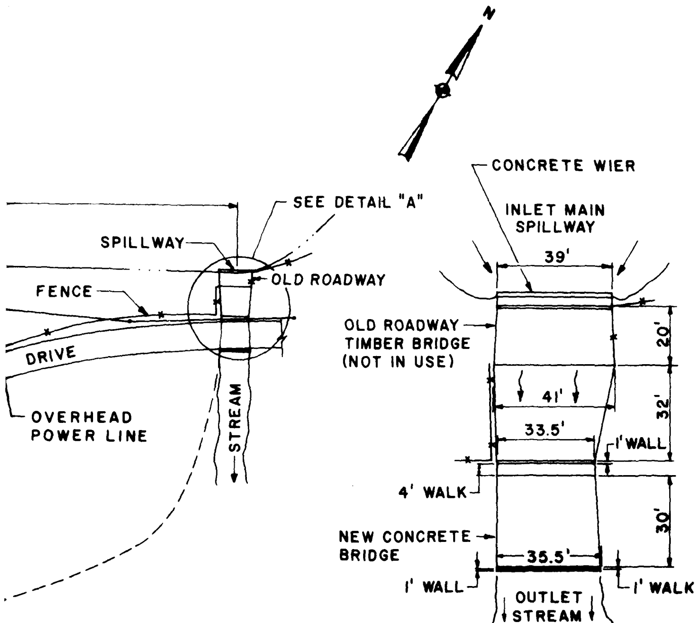
DETAIL "A" SCALE: 1" = 30'
