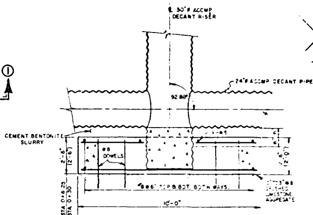
SECTION ①-①
