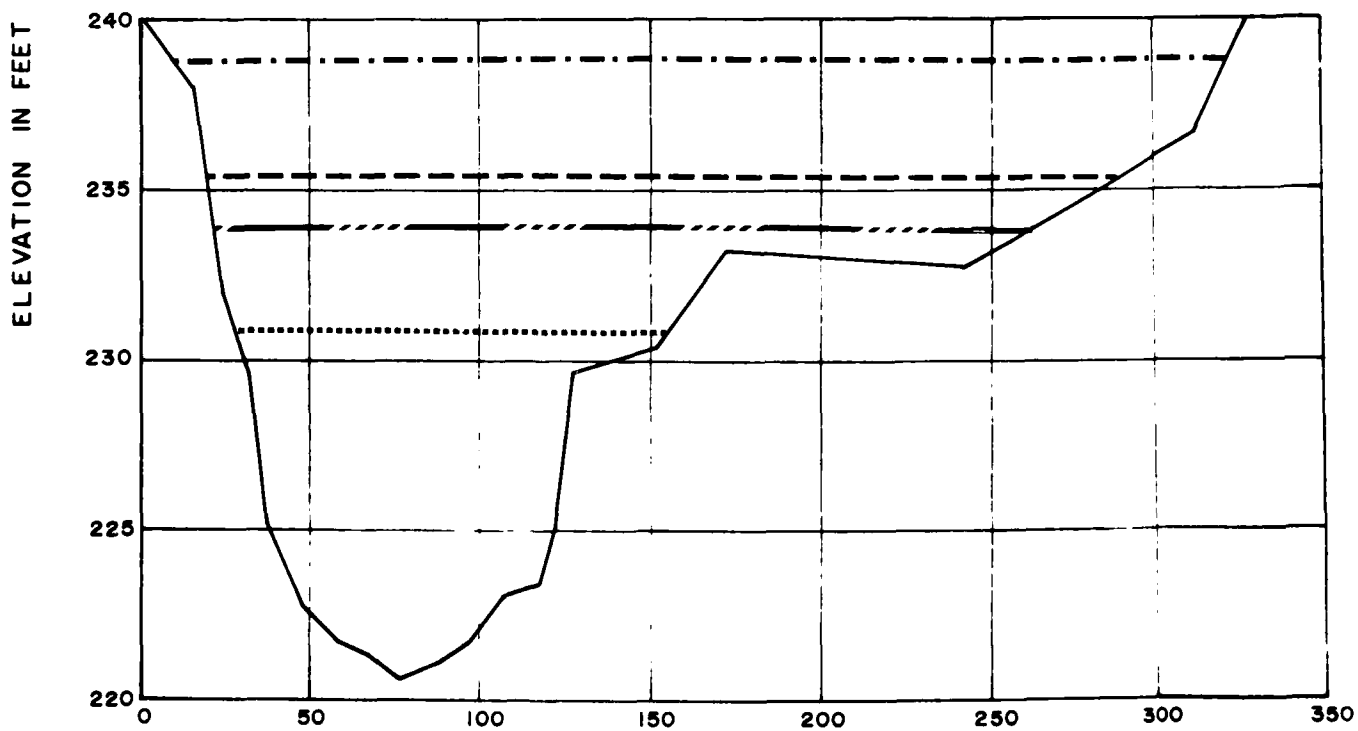
CROSS SECTION NO. 5 STA. 160 + 60
