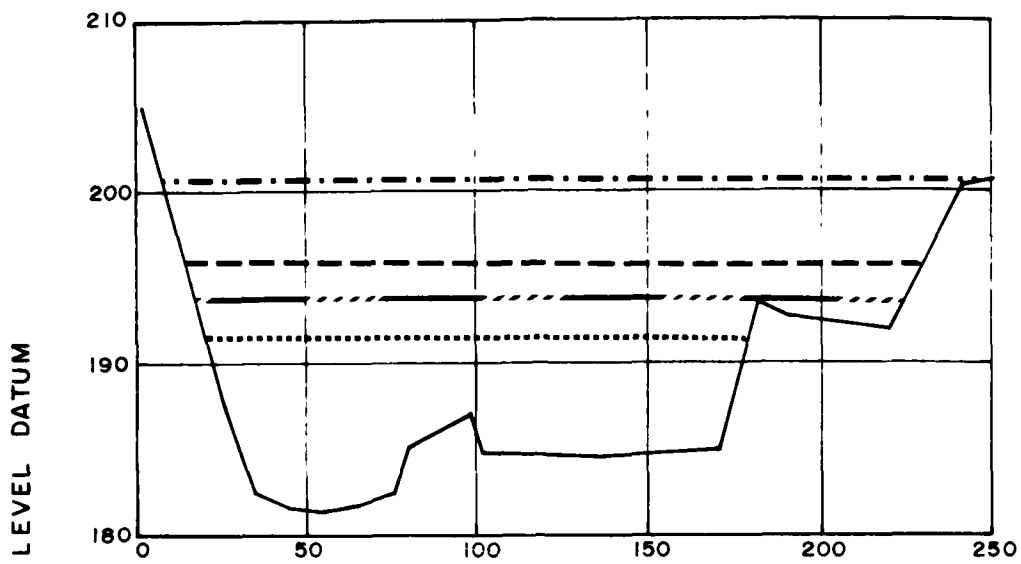
CROSS SECTION NO. 2 STA. 24 + 75
