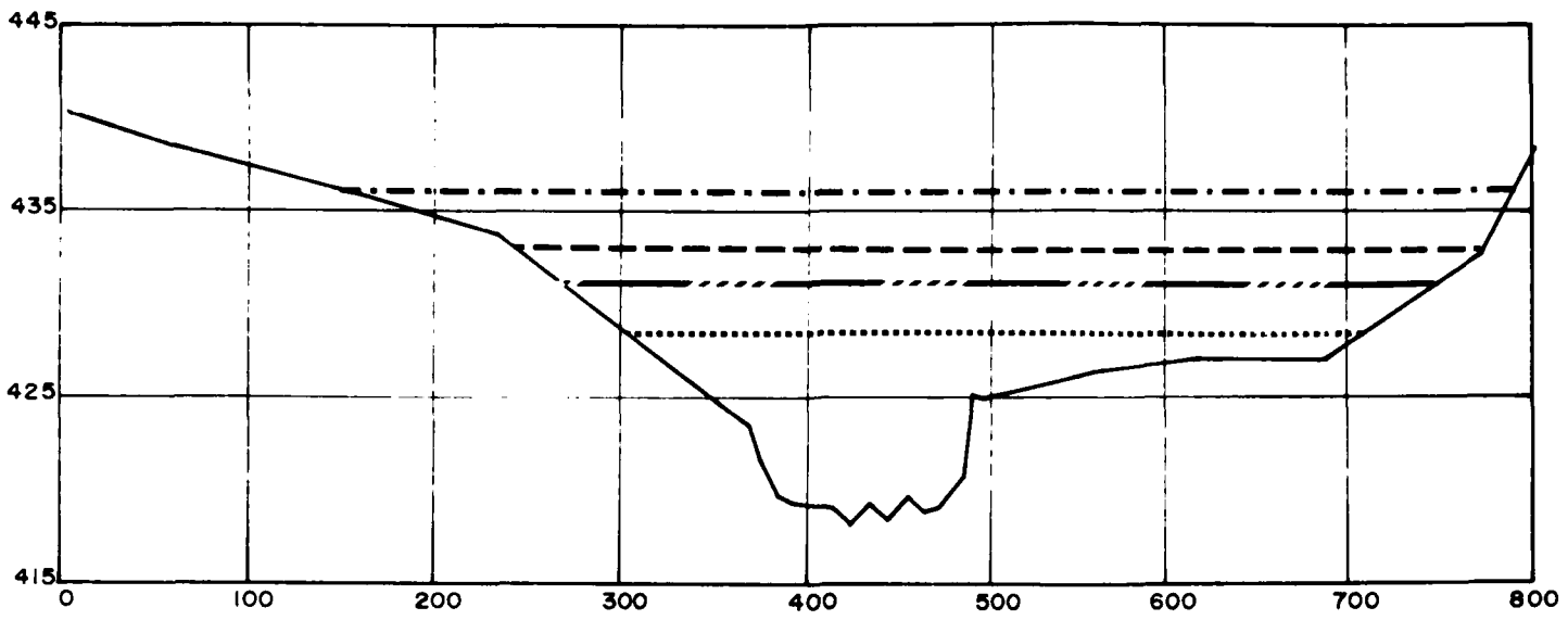
CROSS SECTION NO. 11 STA. 436 + 35
