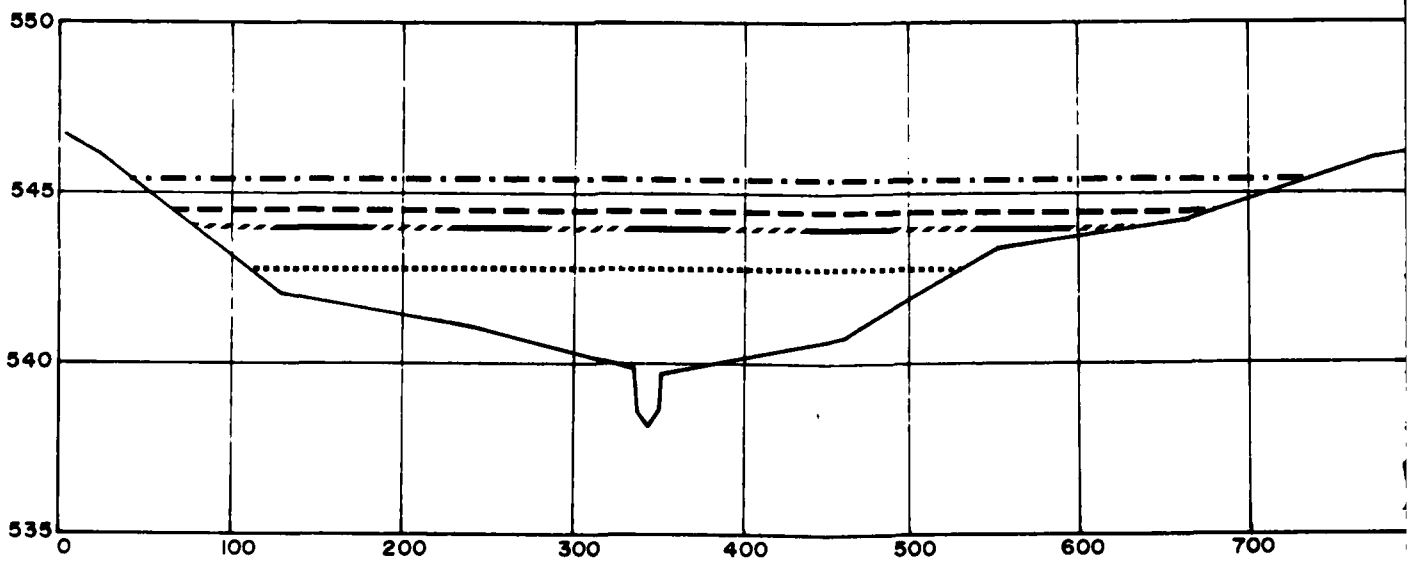
CROSS SECTION NO. 17 STA. 750 + 60
