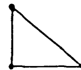
(i) linear element
