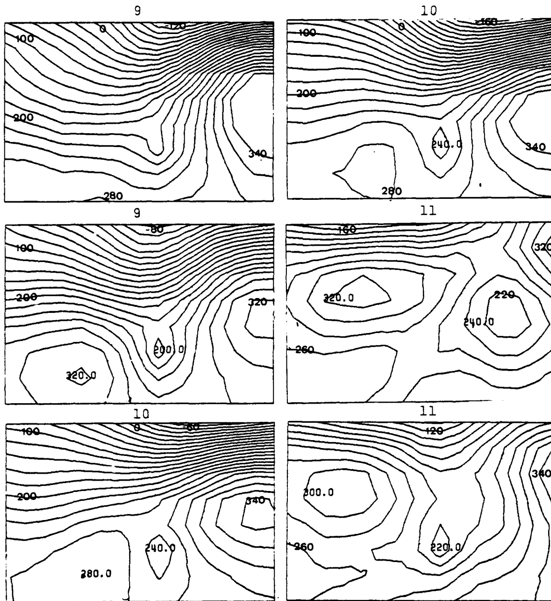
Fig. D1. cont. Examples of map types 9-11.
