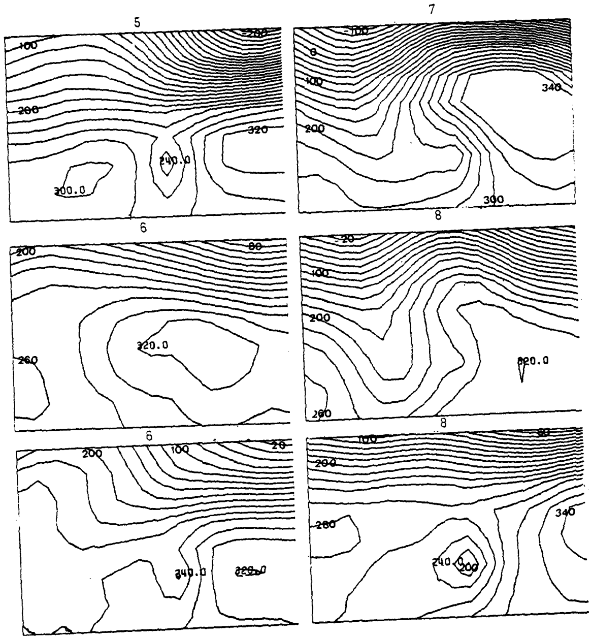
Fig. D1. cont. Examples of map types 5-8.
