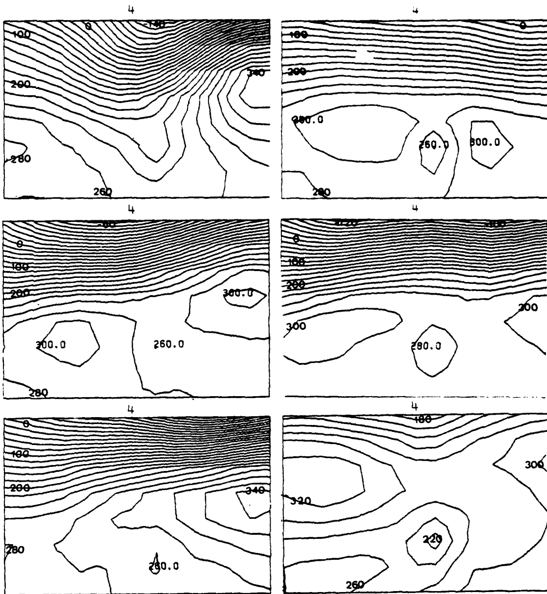
Fig. D1. cont. Examples of map type 4.
