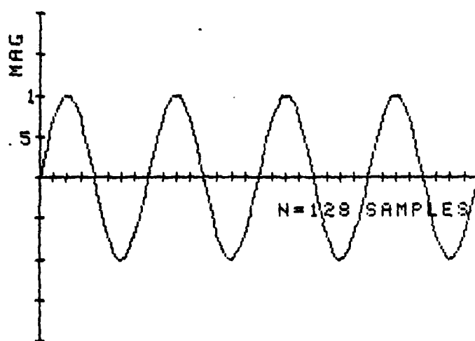
Fig. 4.18. Reference Input
