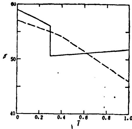
图6 IV 面转面气流角沿通道中线的变化 中弧线—— 计算结果——
