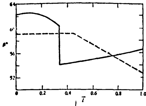
图5 II 面转面气流角沿通道中线的变化 中弧线—— 计算结果——
