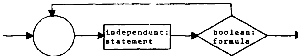
DOUNTIL
