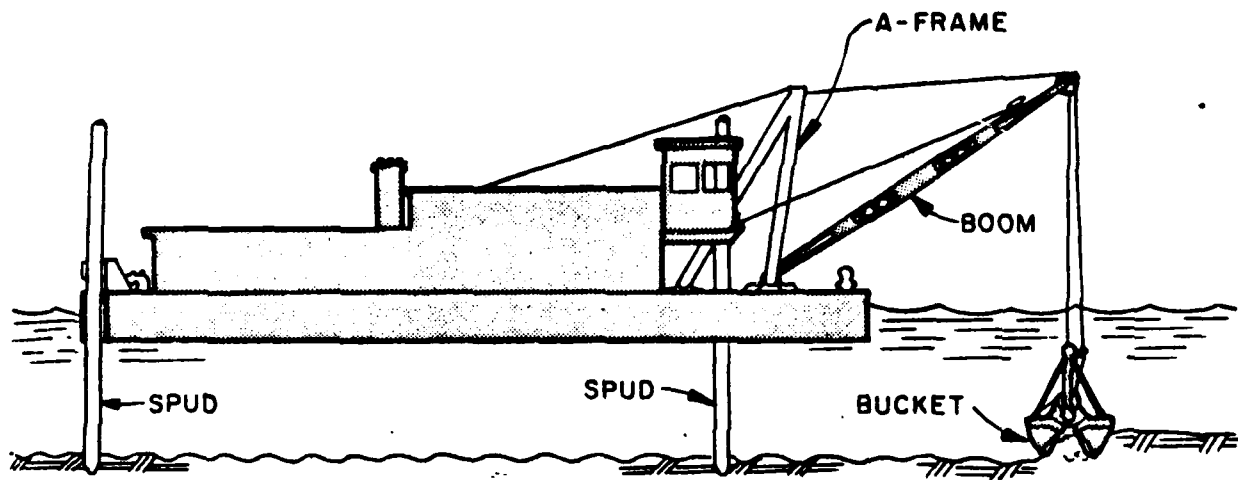
GRAB DREDGE
