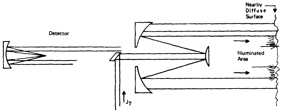
(a) Actual Mirror Configuration
