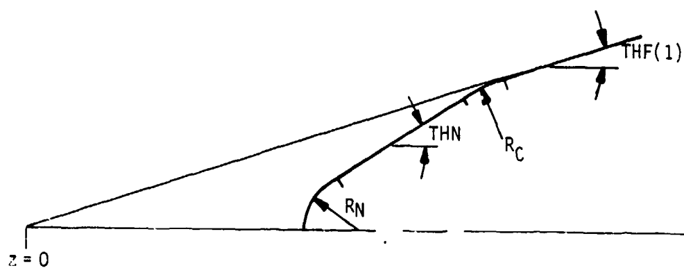
b.) BICONIC NOSETIP
