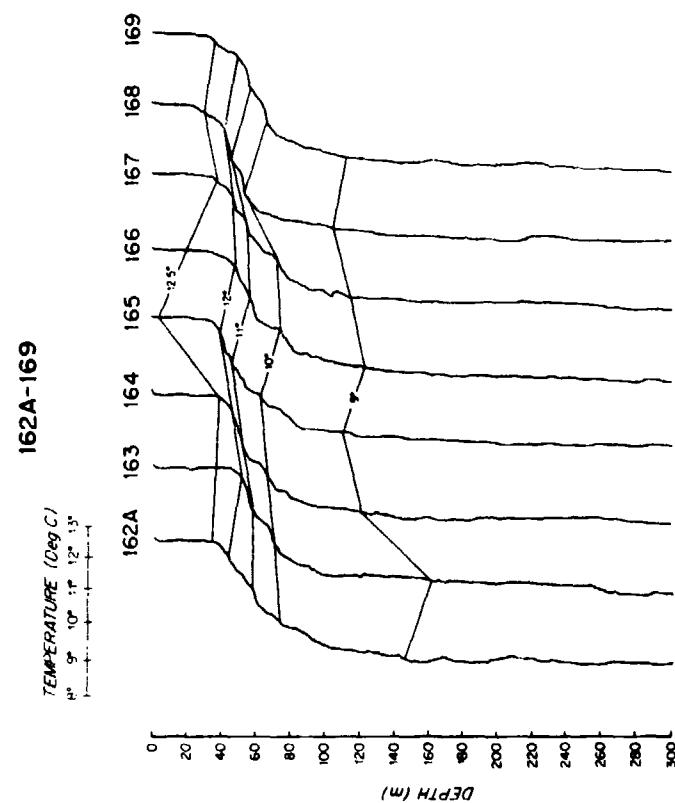
XBT Section 17.
