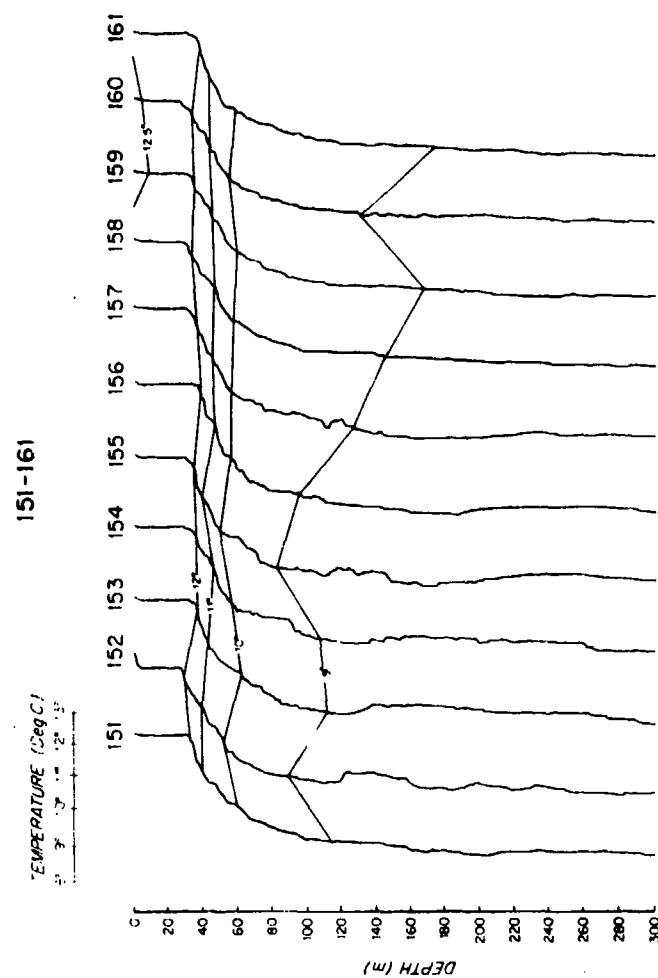
XBT Section 16.
