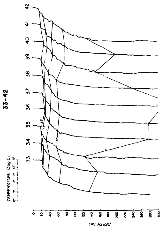
XBT Section 3.
