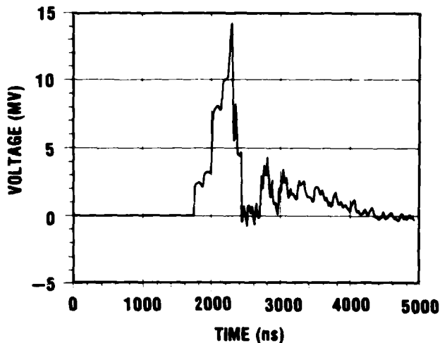
(d) OUTPUT SWITCH, S 2 (MARX SIDE)
