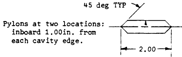
d. Store Pylon
