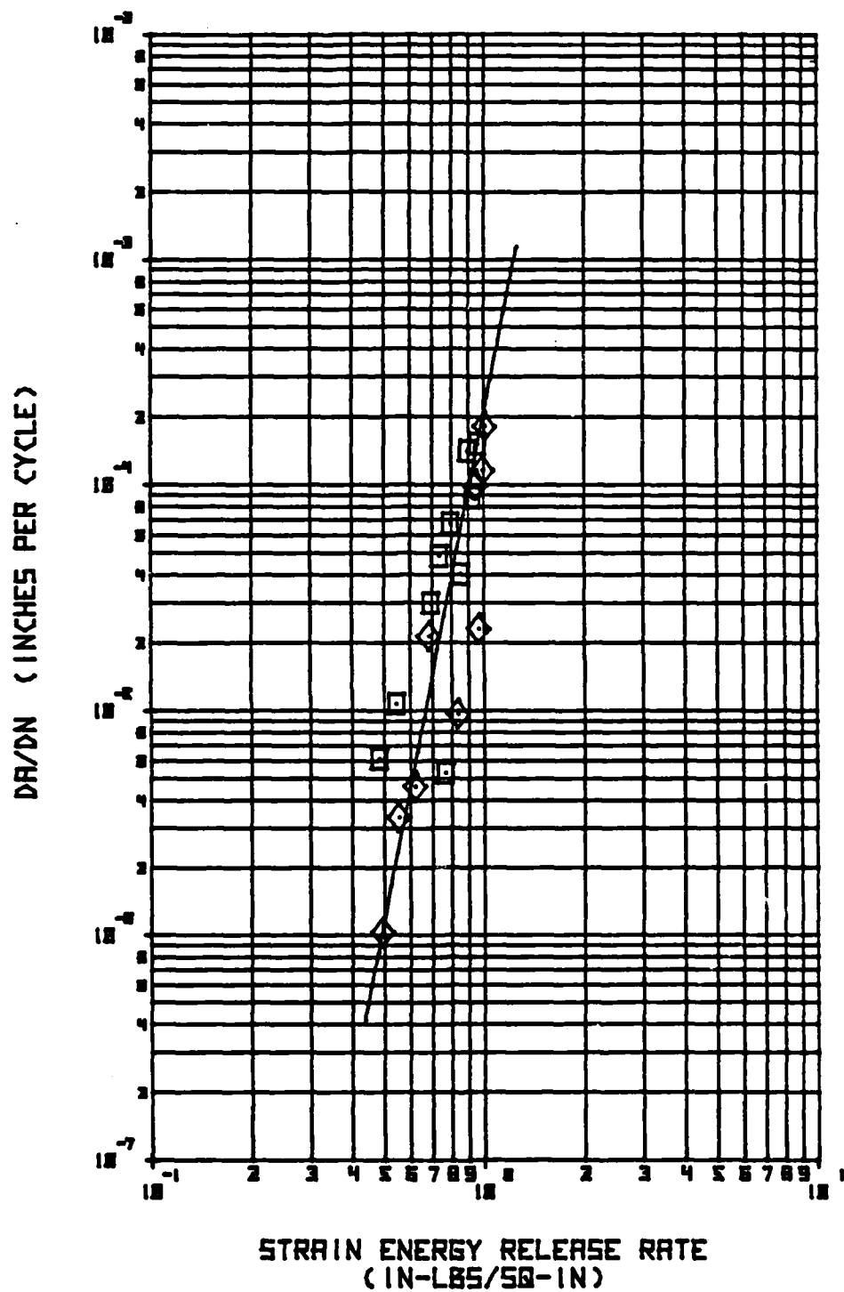
Figure C-6 Test E1RWF of Specimen E1-5-4
