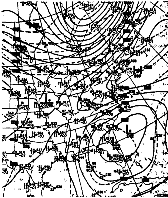
Figure 17. 29/00Z 850-mb Analysis.
