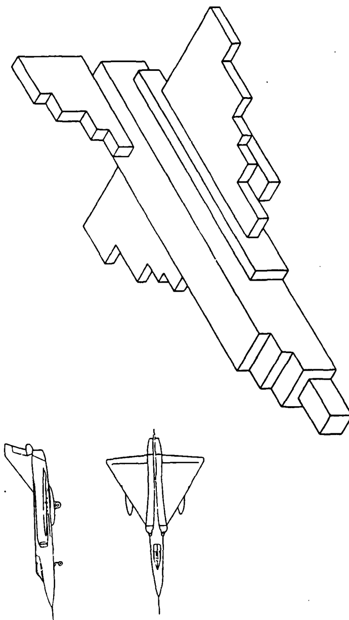
T3DFD MODEL OF F106B
