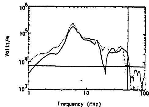
Fig. 24. T.P. 382, Q(\omega) , E \parallel Fuselage.
