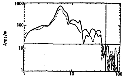
Fig. 22. T.P. 382, J_A(t) , E \parallel Fuselage.
