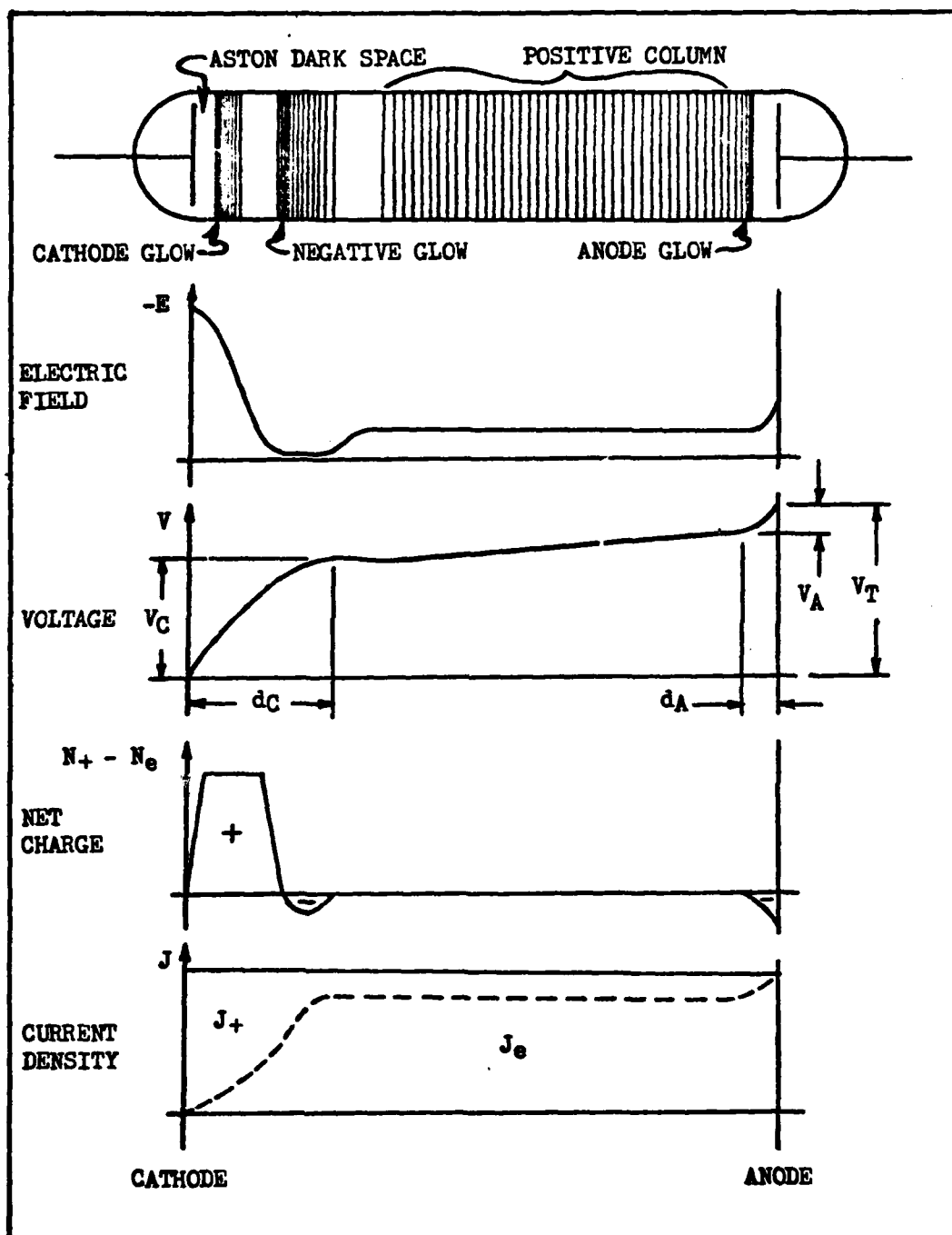
Figure 2. Glow Discharge Parameter Profile
