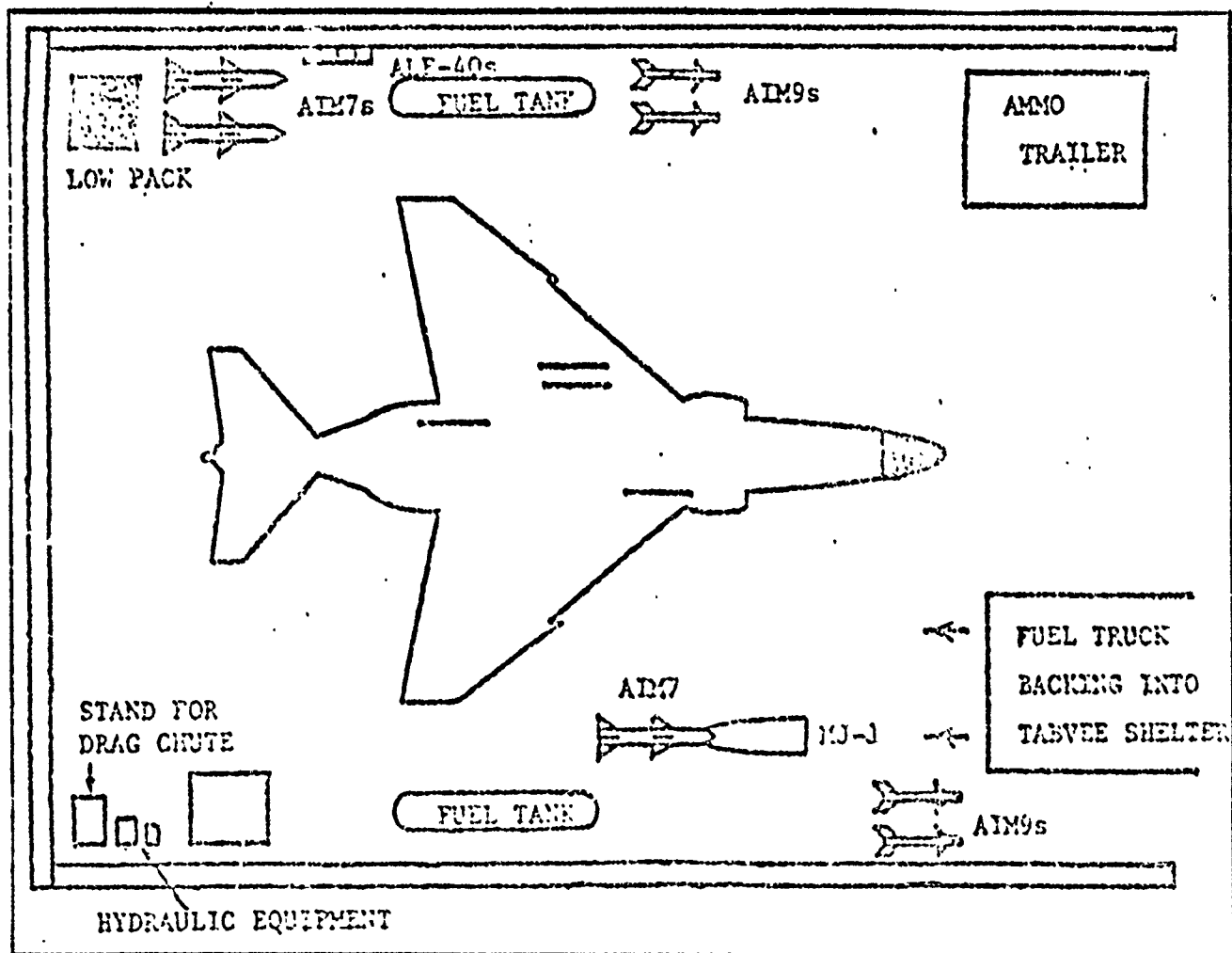
Fig. 3 TABVEE Shelter
