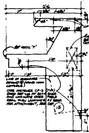
END ELEVATION (5A)
