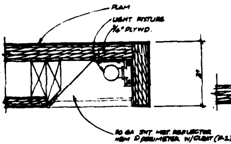
BOOKCASE LIGHT DET. (14) SCALE: 1/8" = 1"
