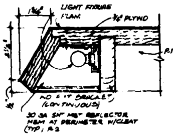
LIGHT FIXT. DETAIL (7) SCALE: 1/8" = 1"
