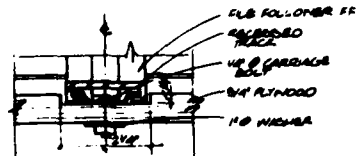
FILE FOLLOWER DET. (10) SCALE: 1/8" = 1"
