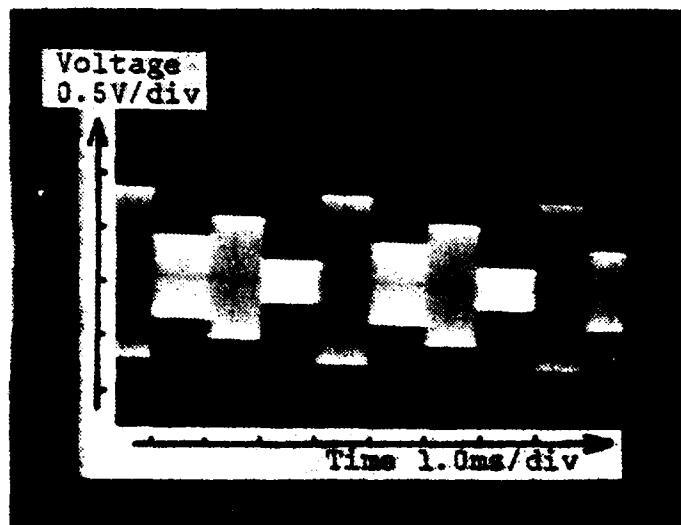
Fig. 3.7. 4-Amplitude Modulator Output
