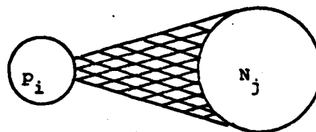
(c) z_{ij} ( i \neq j )
