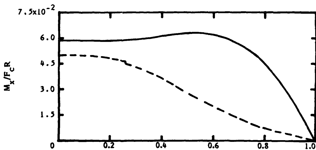
(d) Twisting moment (magnitude).
