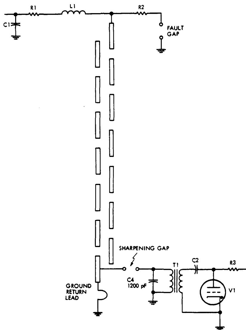
FIG. 9. BOTTOM TRIGGERING
