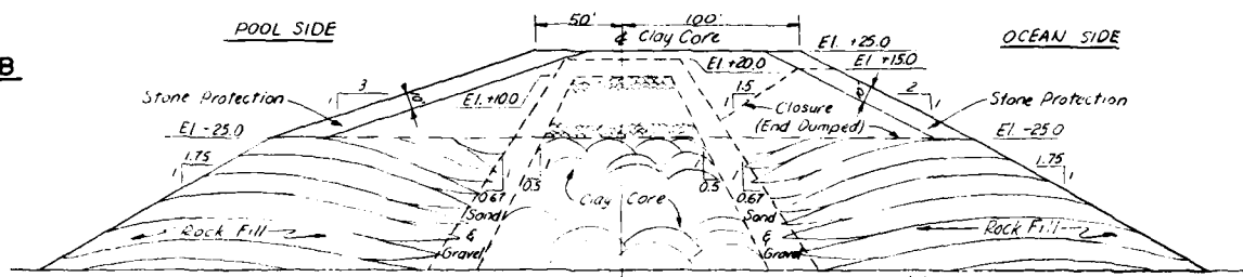
SECTION B SCALE: 1" = 40'
