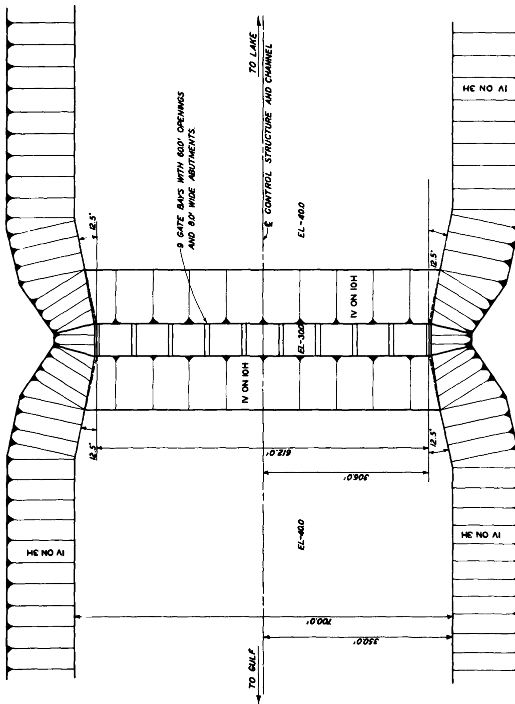
Figure 5. Chef Menteur structure
