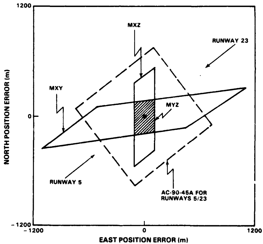
b) Error Parallelograms
