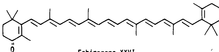
Echinenone XXVI
