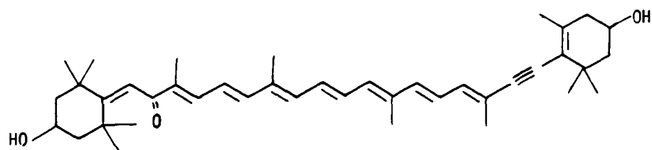
Diadinochrome X
