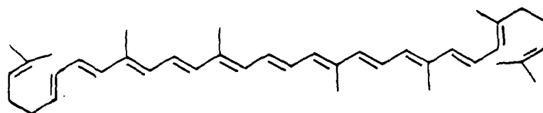
Lyconene XLV
