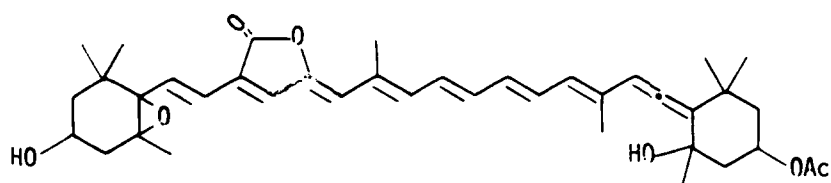
Peridinin V
