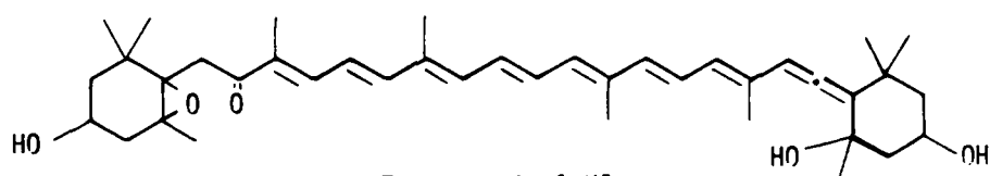
Fucoxanthinol VI
