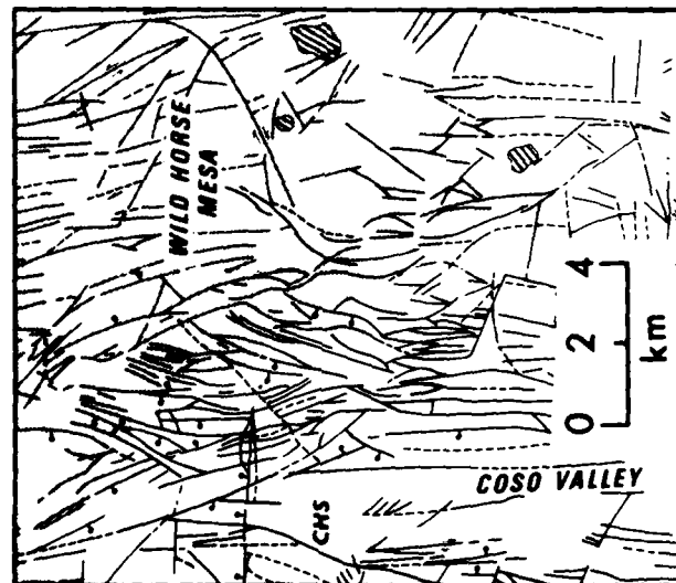
(a) Wild Horse Mesa.
