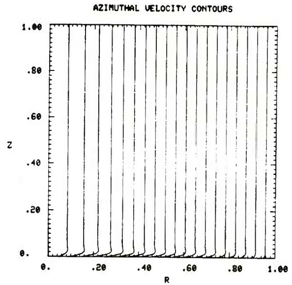
Fig. 4f. Time = 281.25
