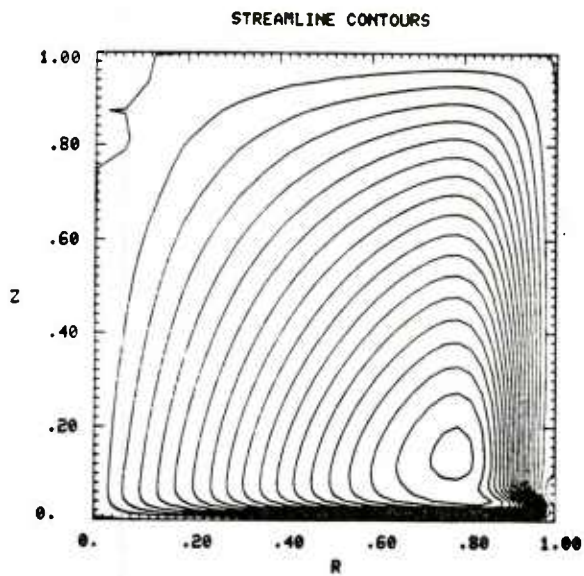
Fig. 5a. Time = 31.25
