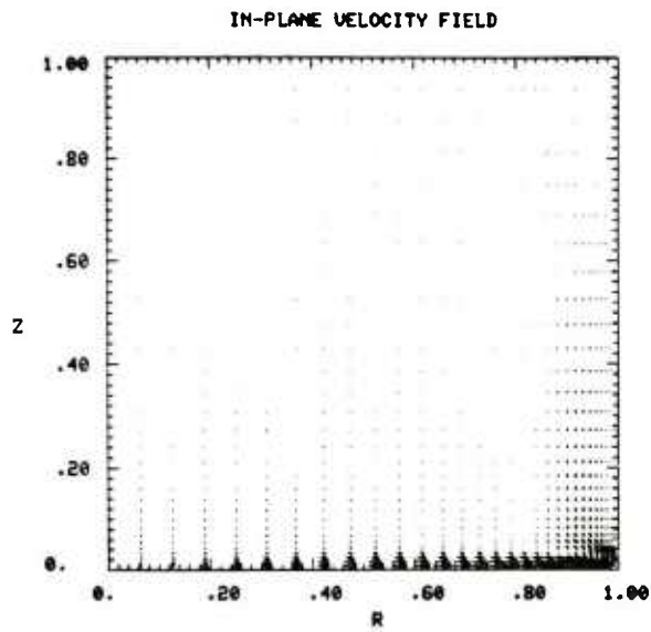
Fig. 3a. Time = 31.25
