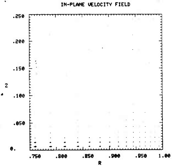
Fig. 3h. Time = 281.25
