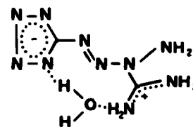
TETRAZENE
