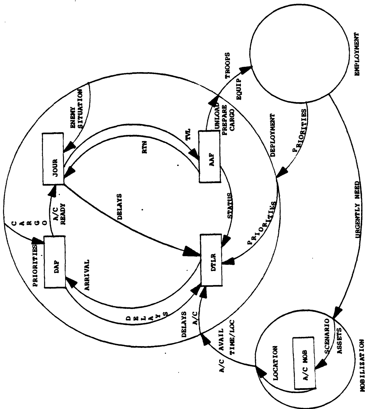
Fig. 4. Air Subarea Interactions
