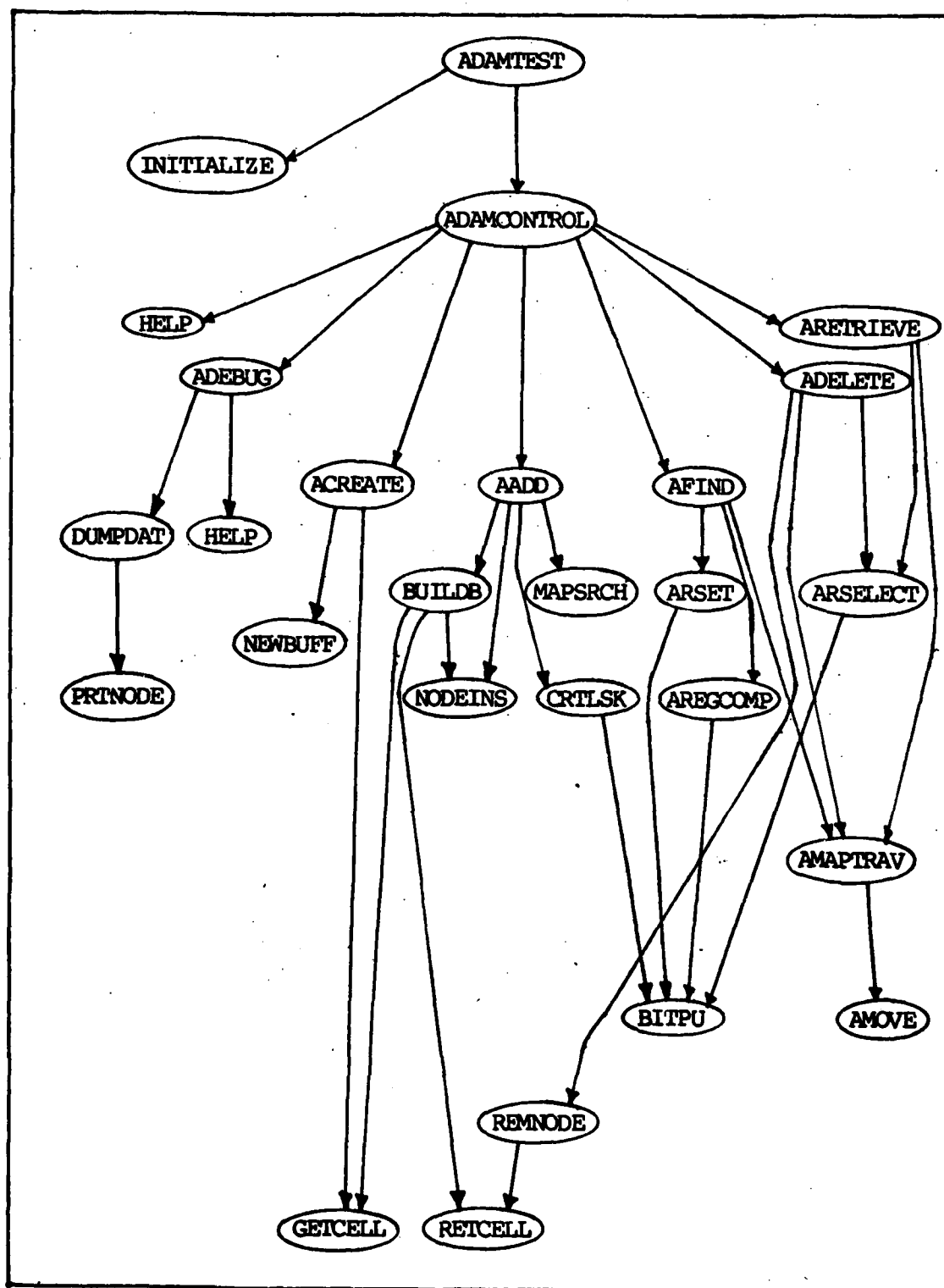
Fig 18. ADAMTEST Hierarchy of Control
