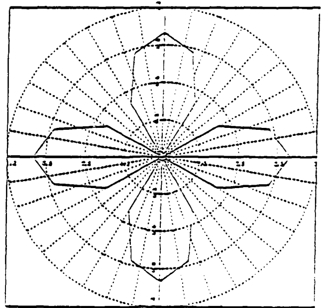
LOVE WAVE
