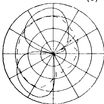
(d) \theta_c=90^\circ , \phi_c=90^\circ , \theta_p=90^\circ
