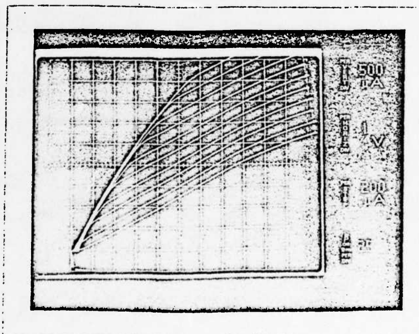
Fig. 4.5f. V_G = 20V .
