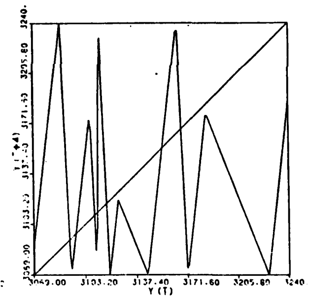
(d) Fourth Iterate
