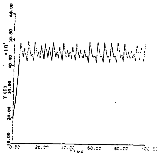
(d) A Sample Chaotic Trajectory
