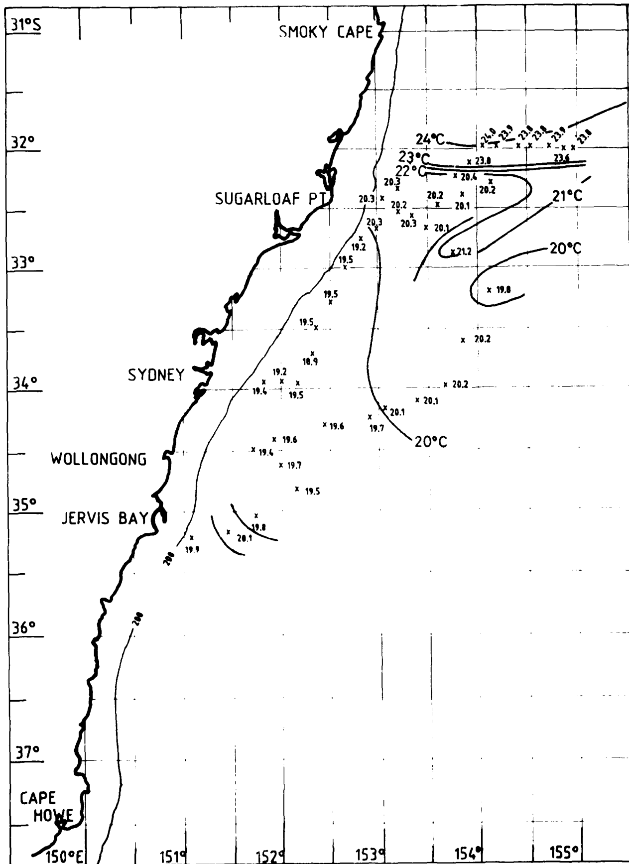
Fig. 26. SST(°C) from Kimbla 16-20 Nov. 81.
