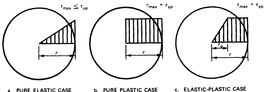
a. PURE ELASTIC CASE
