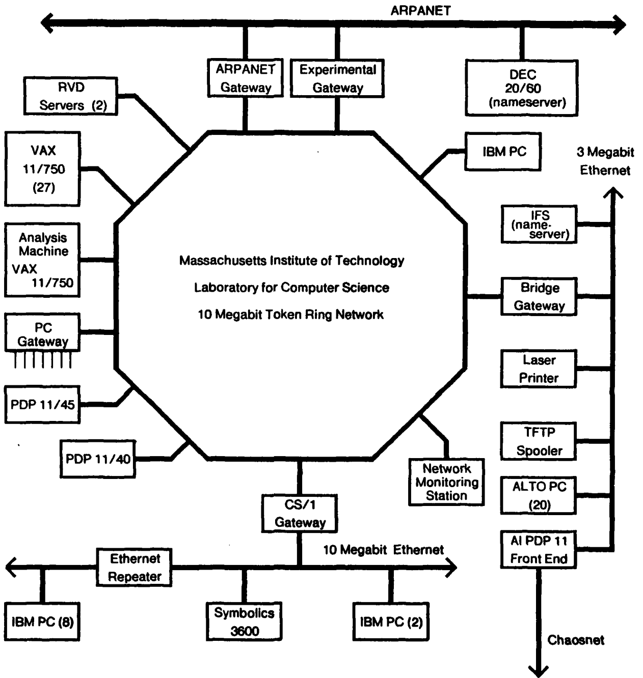
Figure 2-1: The MIT LCS 10 Megabit Ring Network
