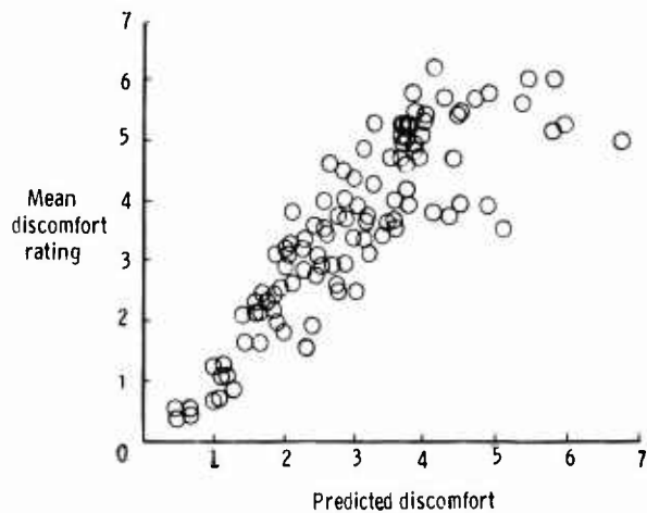
(d) NASA discomfort index; r = 0.914 .
