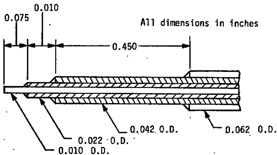
a. Pitot Pressure Probe
