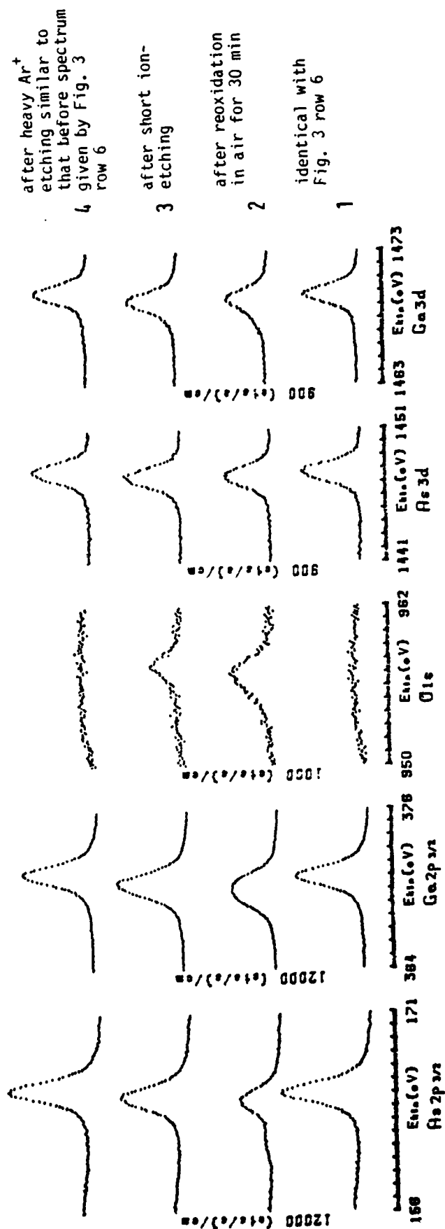
Fig. 4 XPS-spectra
