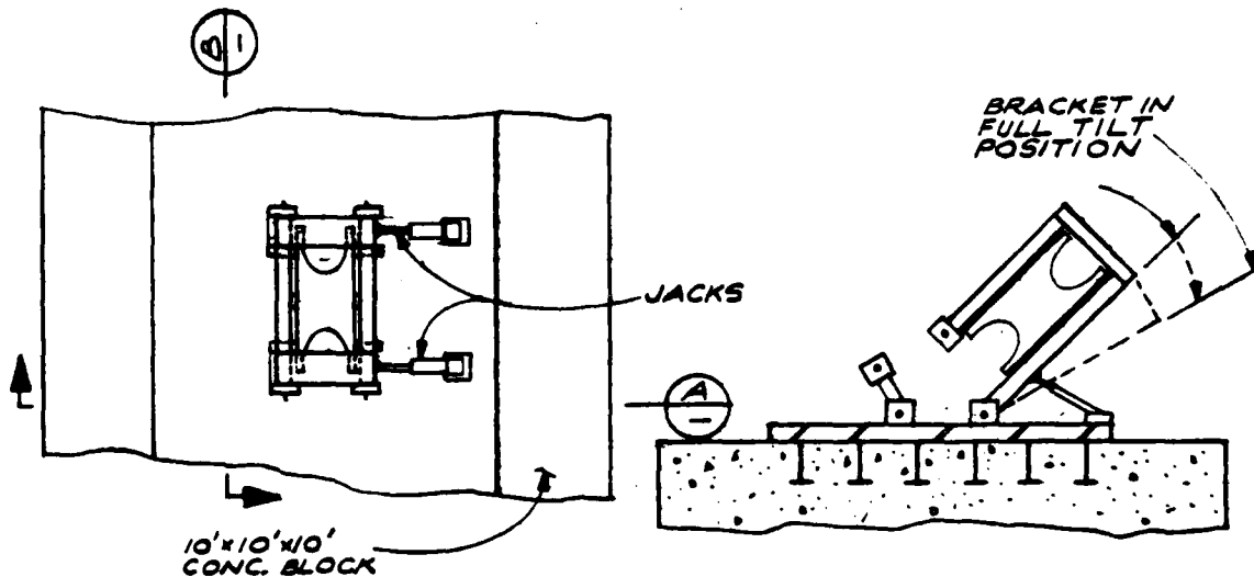
SHEAVE BRACKET IN OPEN POSITION (D)
