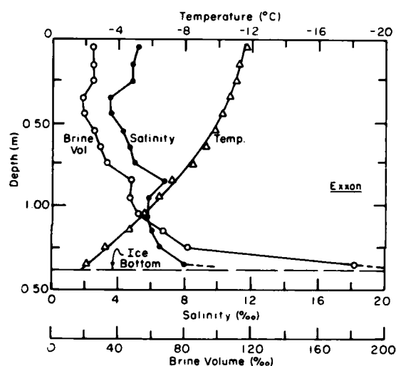
b. Exxon site.
