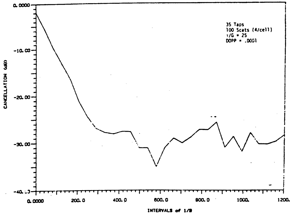
Fig. 27 -- Scatter Cancellor - DOPP = .0001
