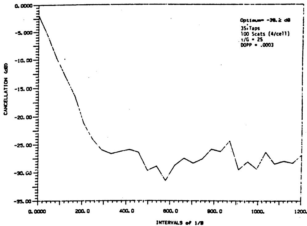
Fig. 28 -- Scatter Cancellor - DOPP = .0003
